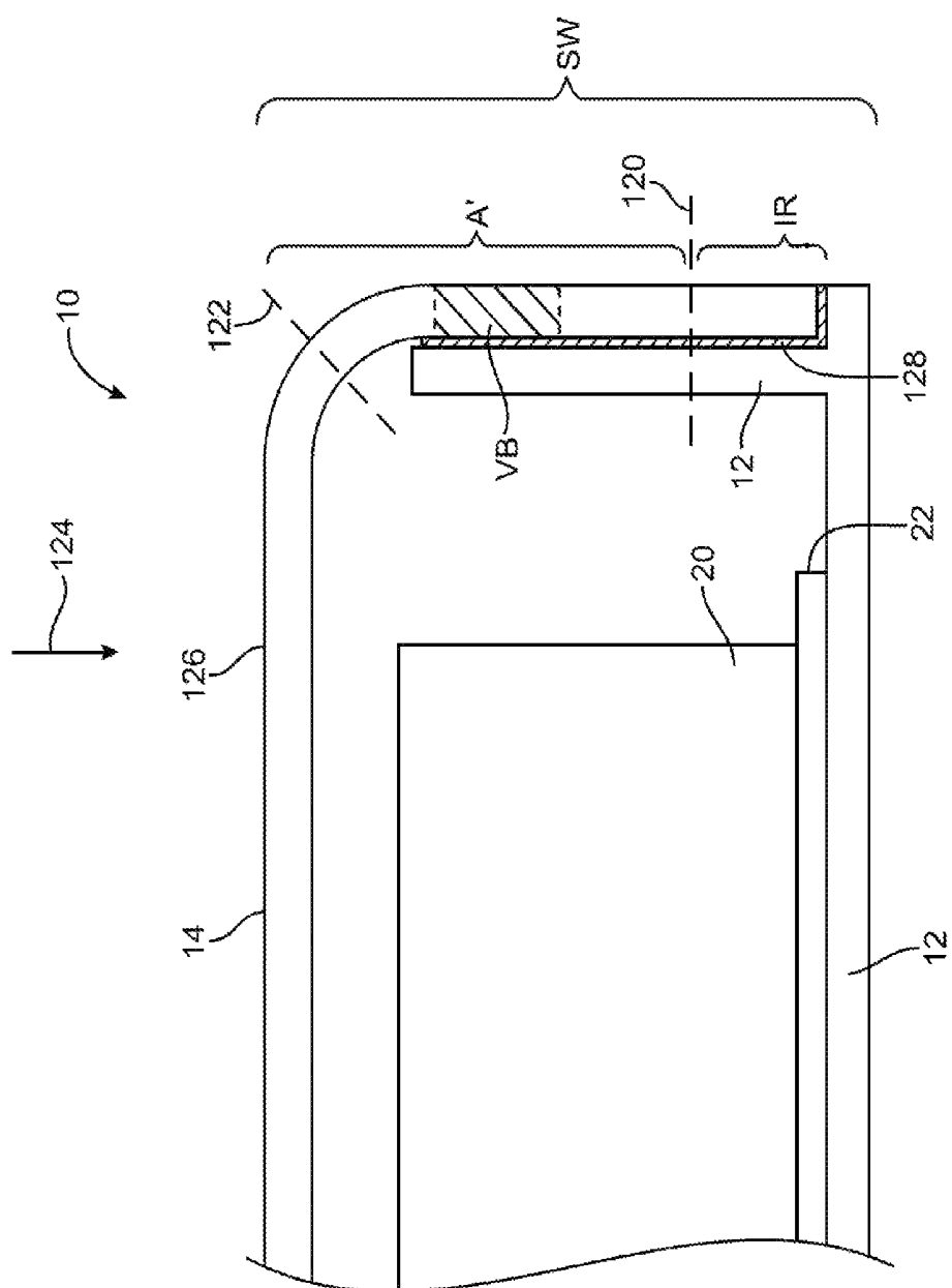
FIG. 34
